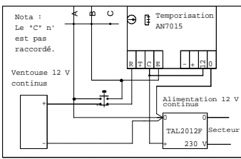
Système GACHE à RUPTURE et VENTOUSE
