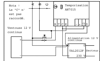
Système GACHE à RUPTURE et VENTOUSE
