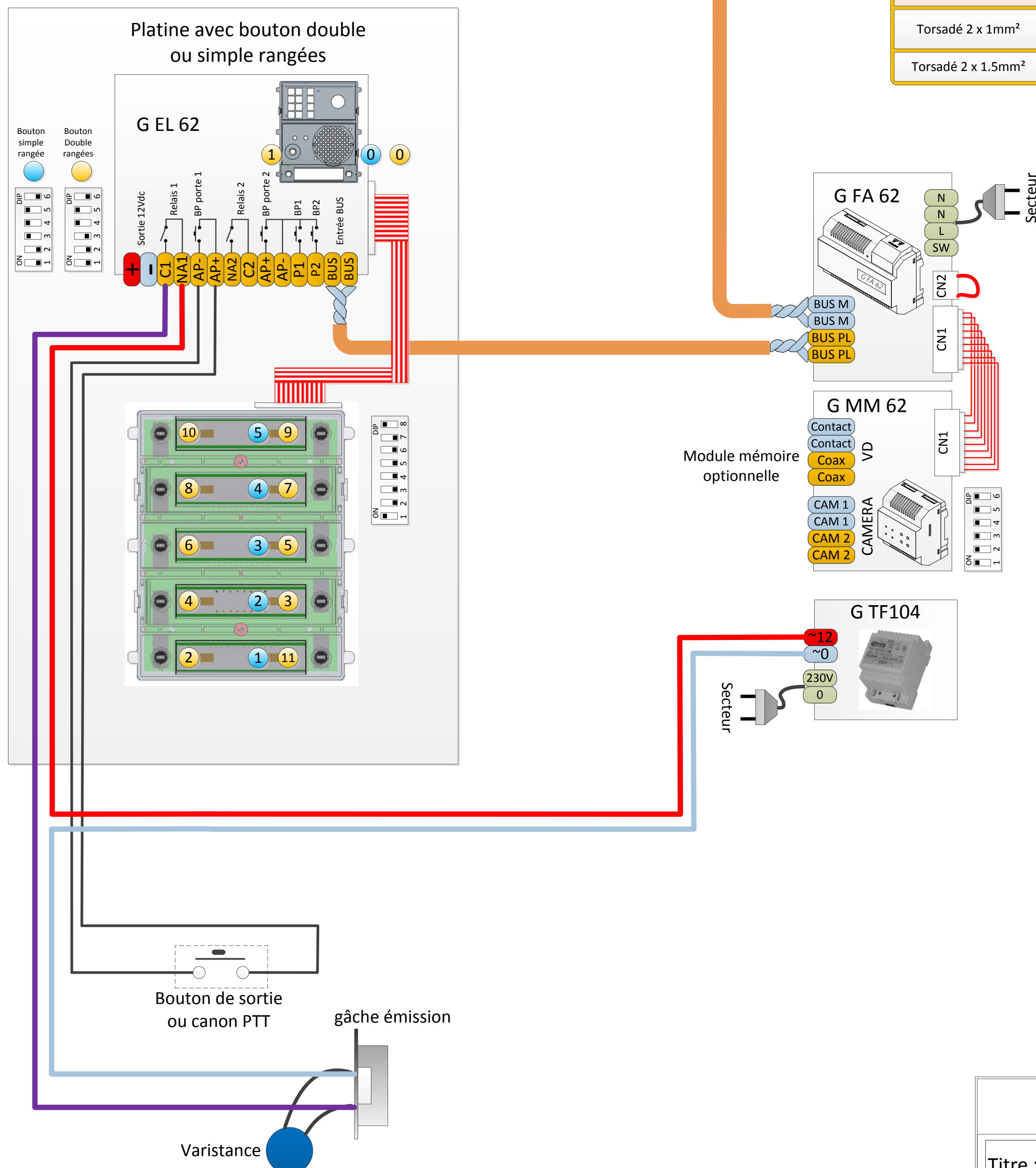
Type de câble pour une quantité > 20 moniteurs
